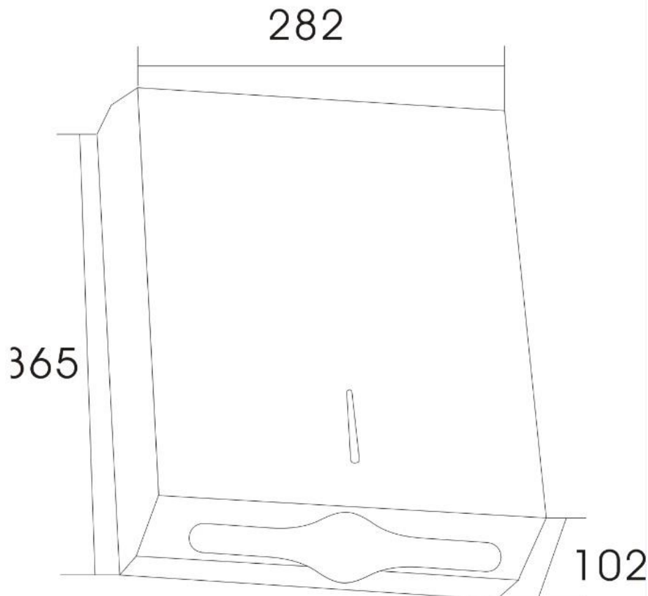
Figura 2: Dimensiones
