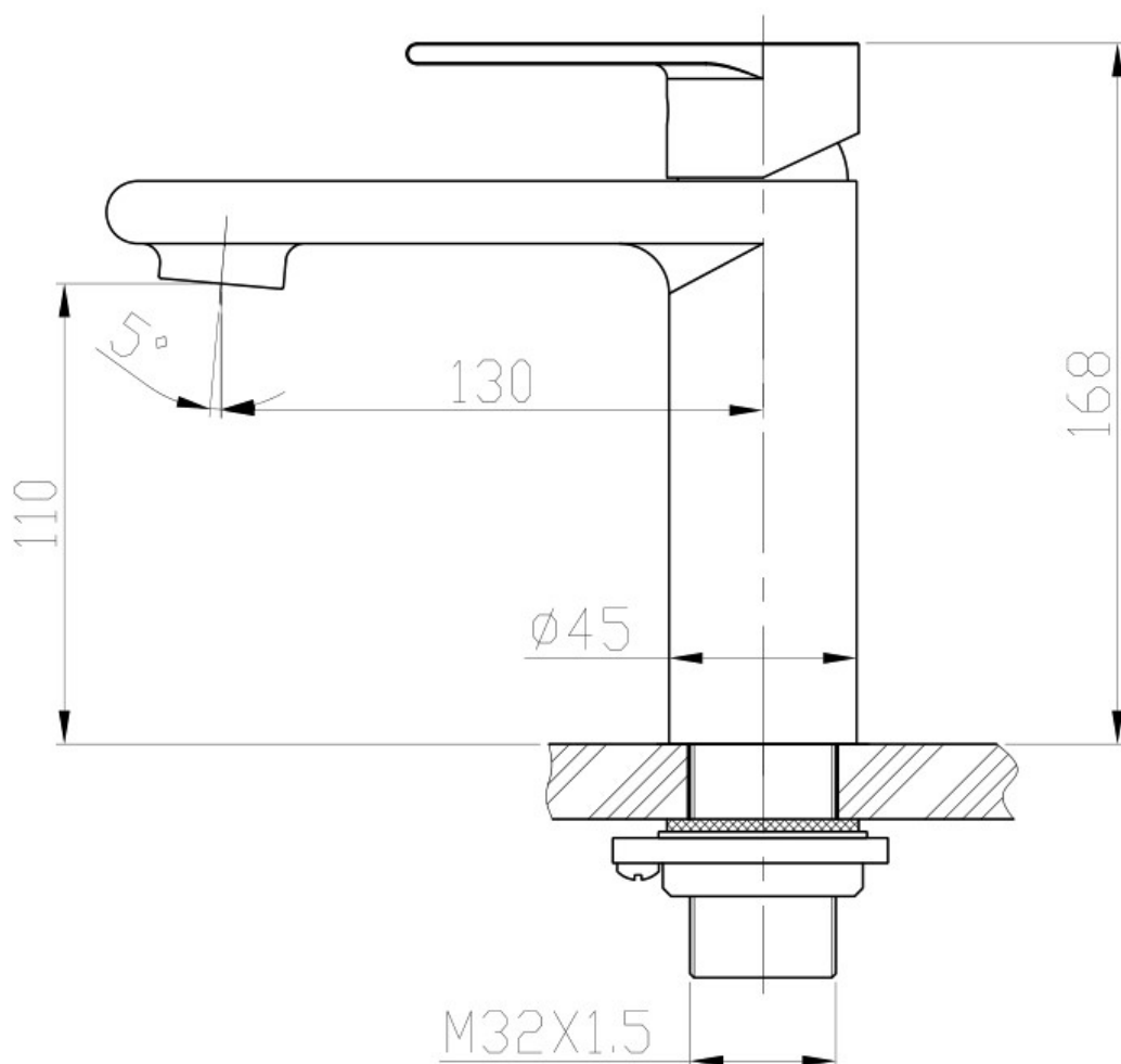
Figura 2: DIBUJO LINEAL
