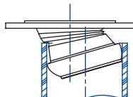
Tubería en Desfasamiento hasta 2.5 cm
