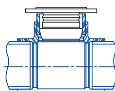
Tubería "T" o codo
